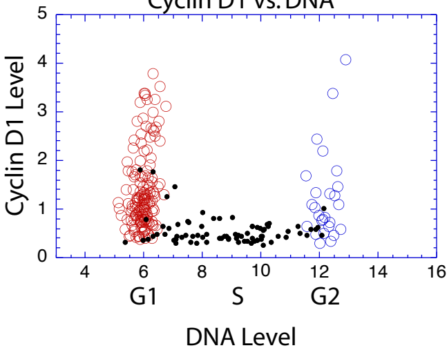
Cyclin D1 vs. DNA
